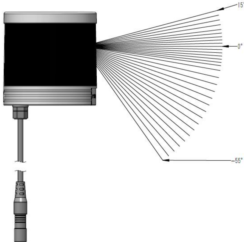
图 13 RS-Helios-5515 俯仰角定义
