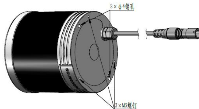
图 5 雷达底部定位销及螺丝示意图
