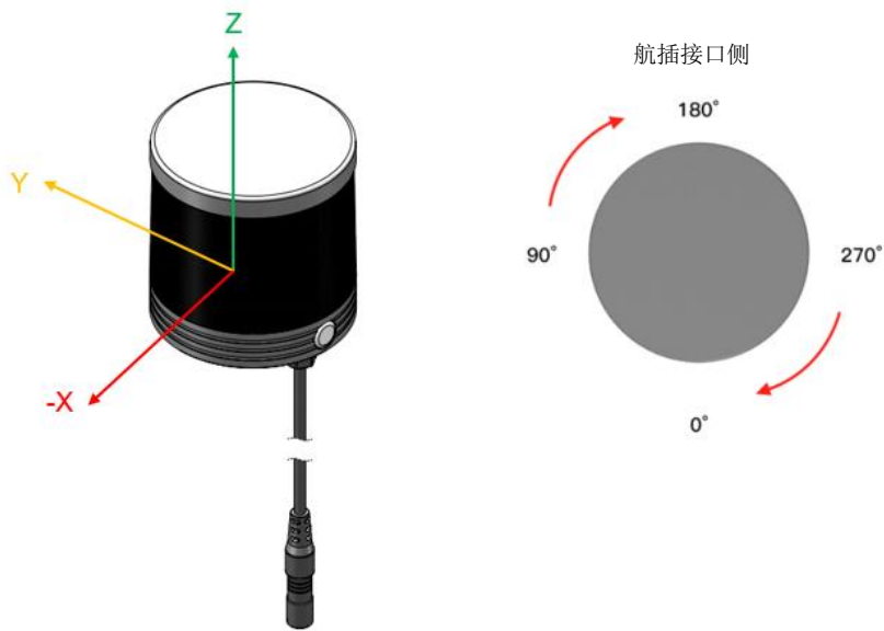
图 1 LiDAR 坐标及旋转方向示意图
