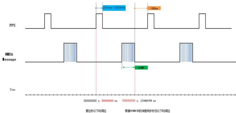
图 9 GPS 时间同步时序图
