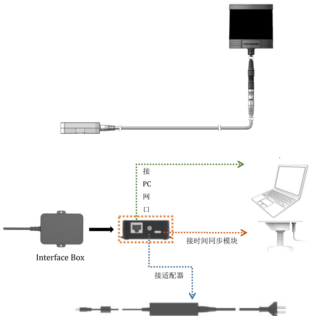
图 6 Interface Box 连接示意图
