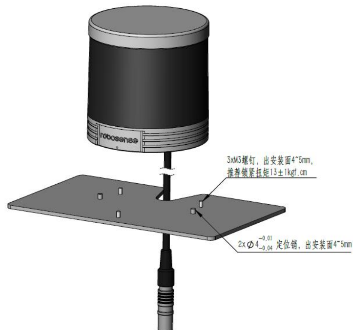
图 4 雷达结构安装示意图
