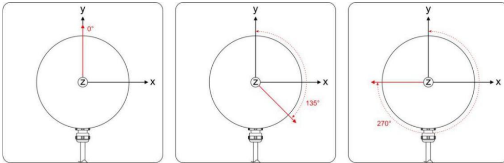
图 8 RS-Helios-5515 不同相位设定示意图
